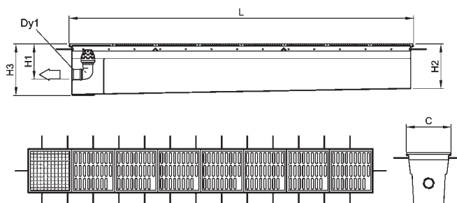
Пескоилоотделители НЕК 5/20...5/80
