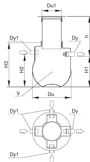
Пескоилоотделители HEK TEL
